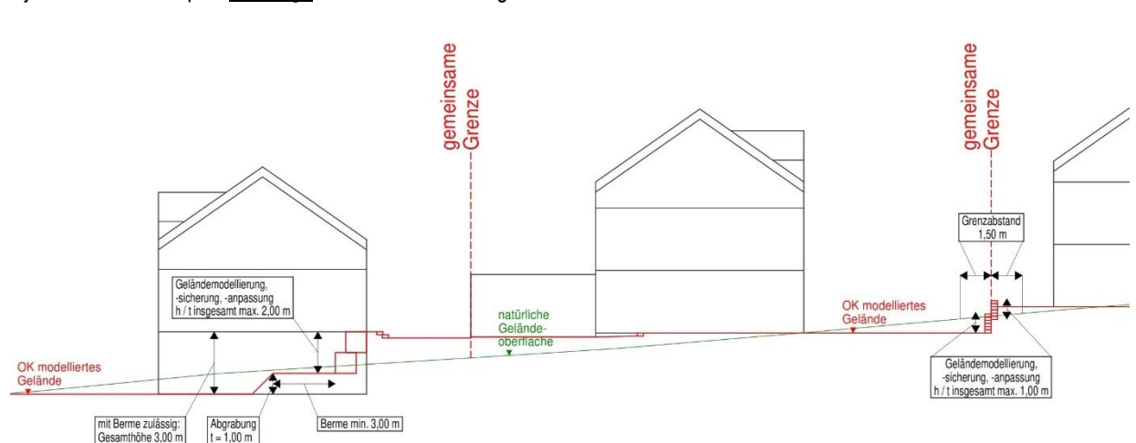
Systemskizze / Beispiel: zulässige Geländemodellierung
