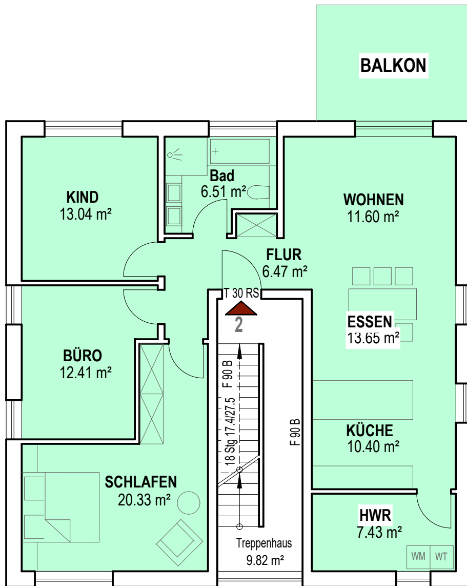
Obergeschoss M 1:100
