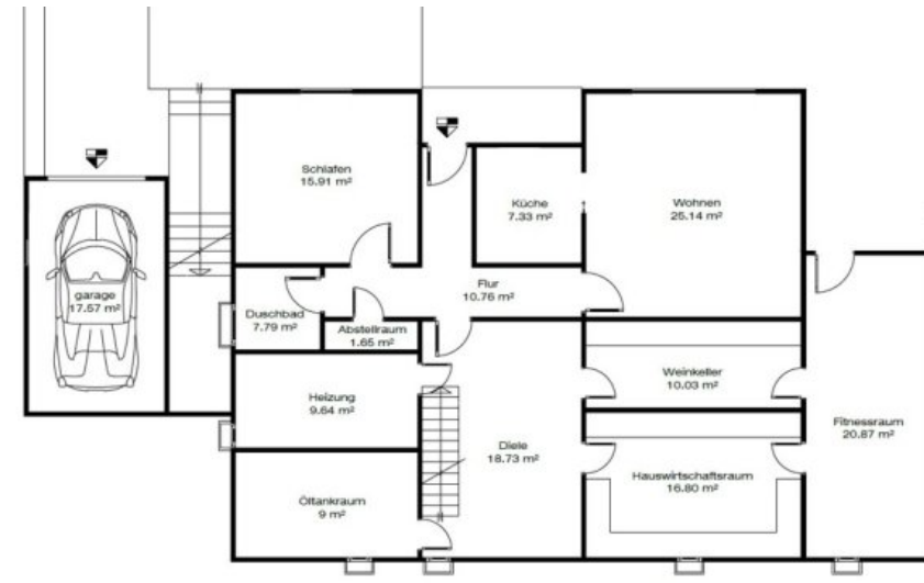
Grundriss Untergeschoss
