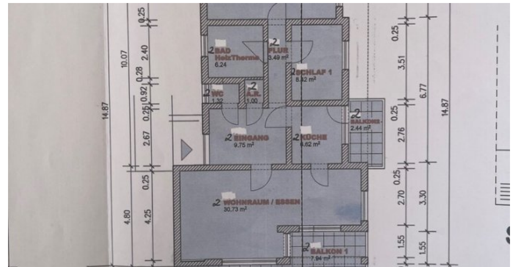
Grundriss OG obere Ebene
