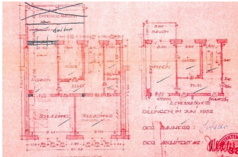
Grundrisse OG 1 und OG 2
