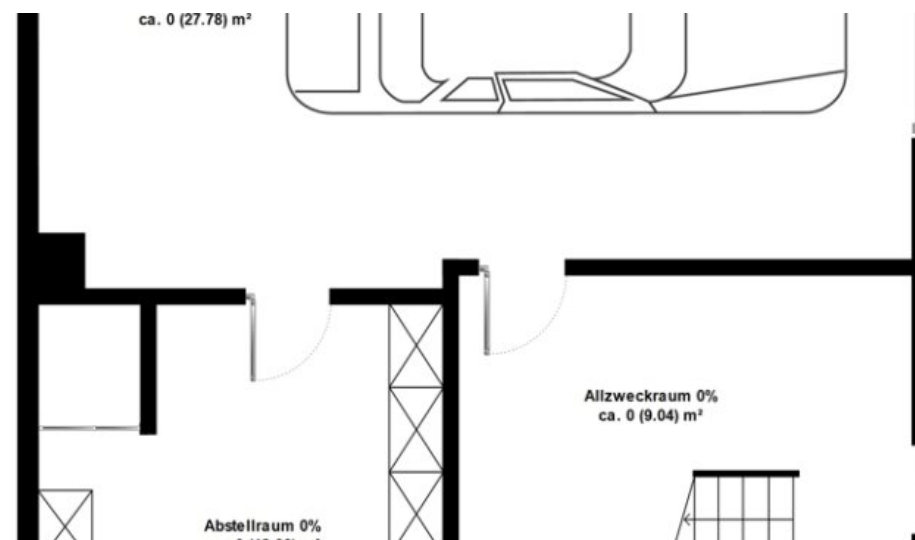
Grundriss KG
