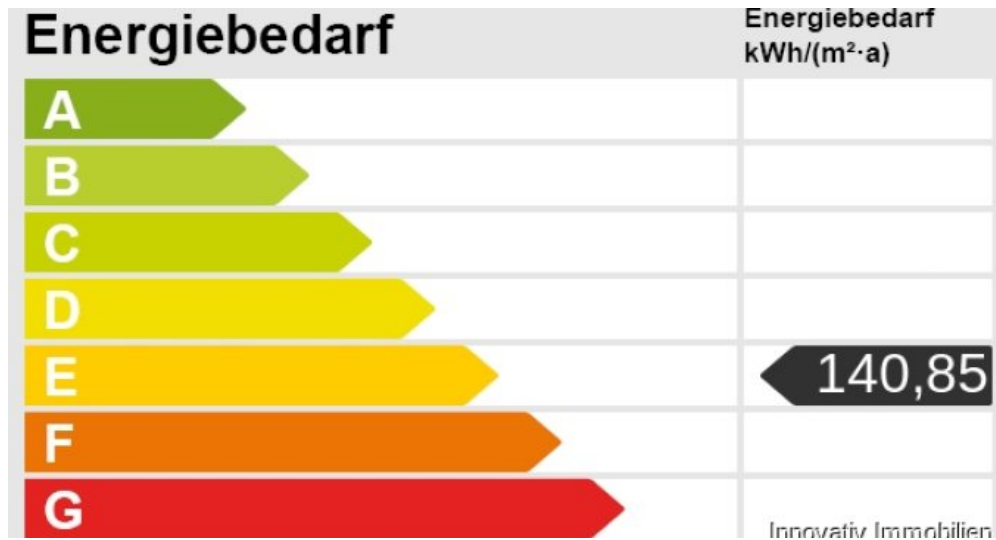
Energieskala
