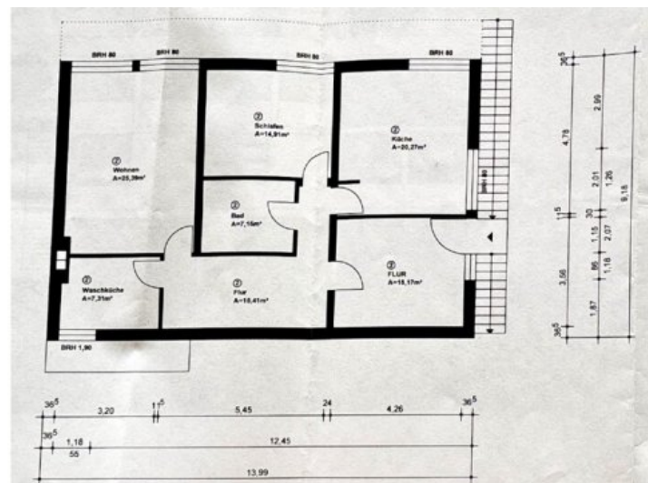
Grundriss WHG 2
