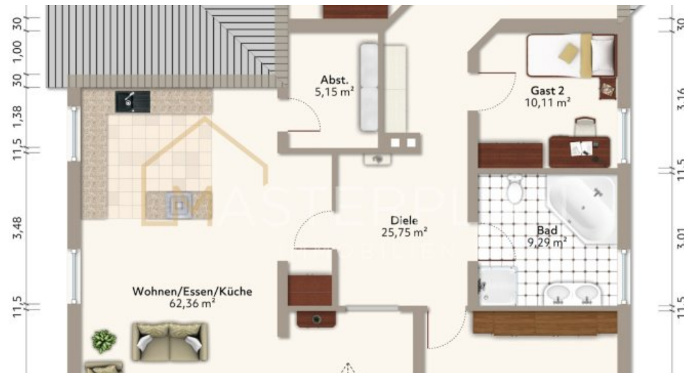
Grundriss WHG 2
