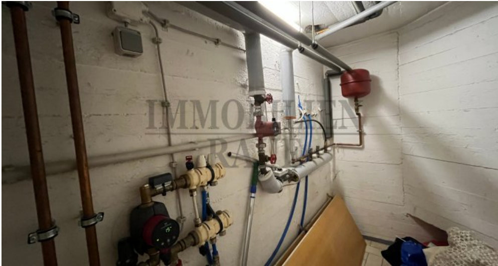
Steuerung Fußbodenheizung (Anbau)
