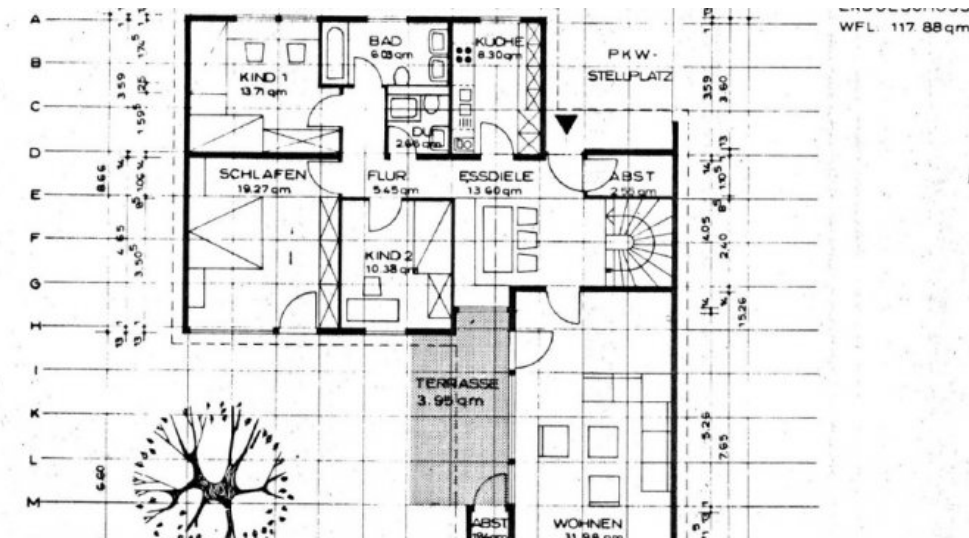
Grundriss EG
