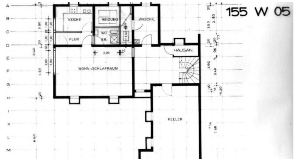
Grundriss UG
