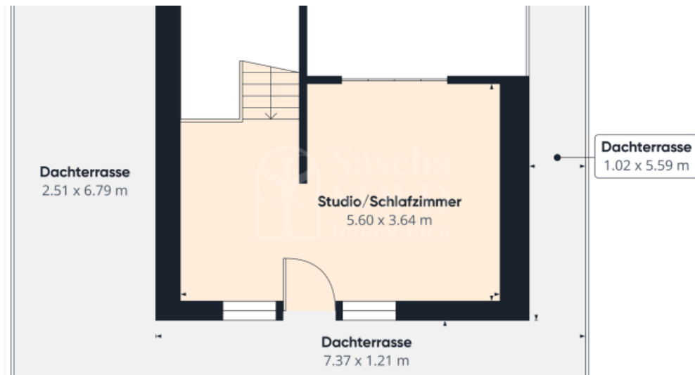
Grundriss - DG
