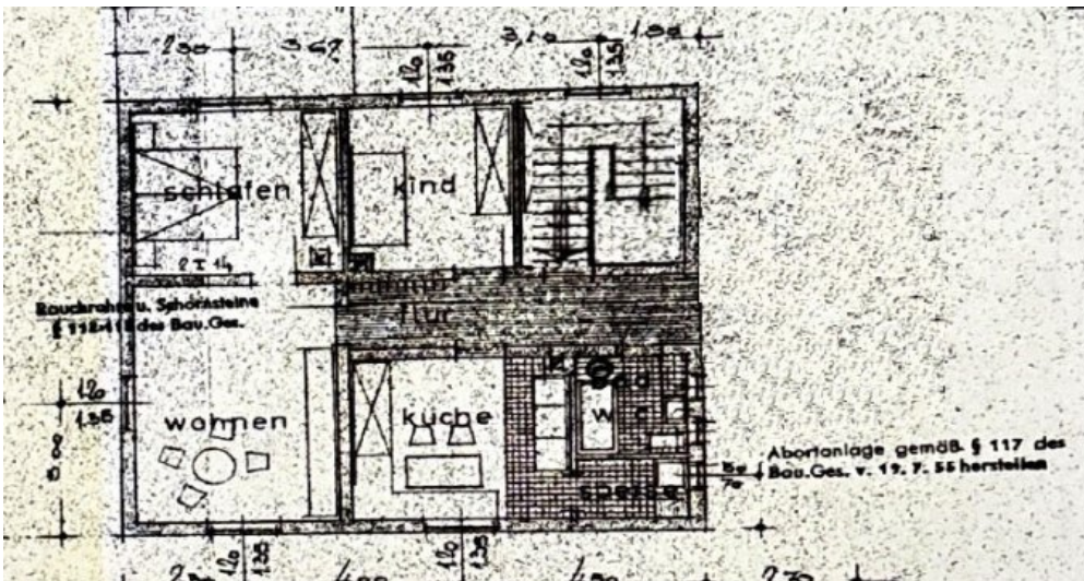
Grundriss OG
