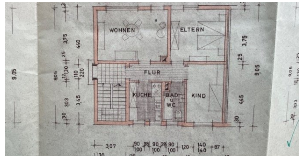
Grundriss Erdgeschoss
