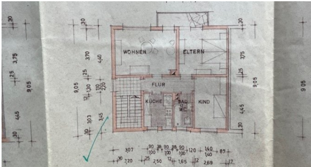
Grundriss Obergeschoss
