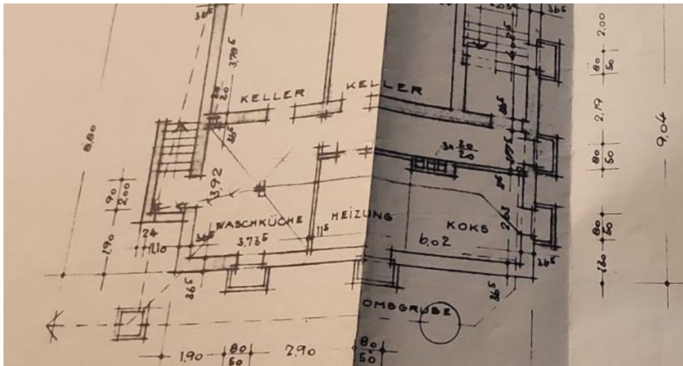
Grundriss Keller
