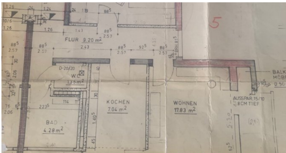
Grundriss WHG 5
