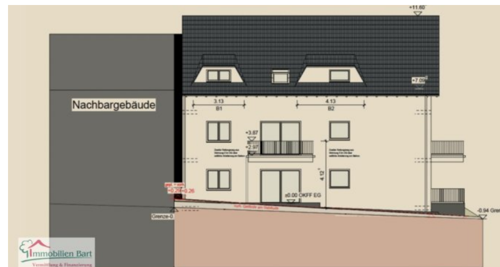
Linke Sietenansicht
