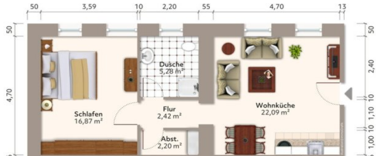
Grundriss
