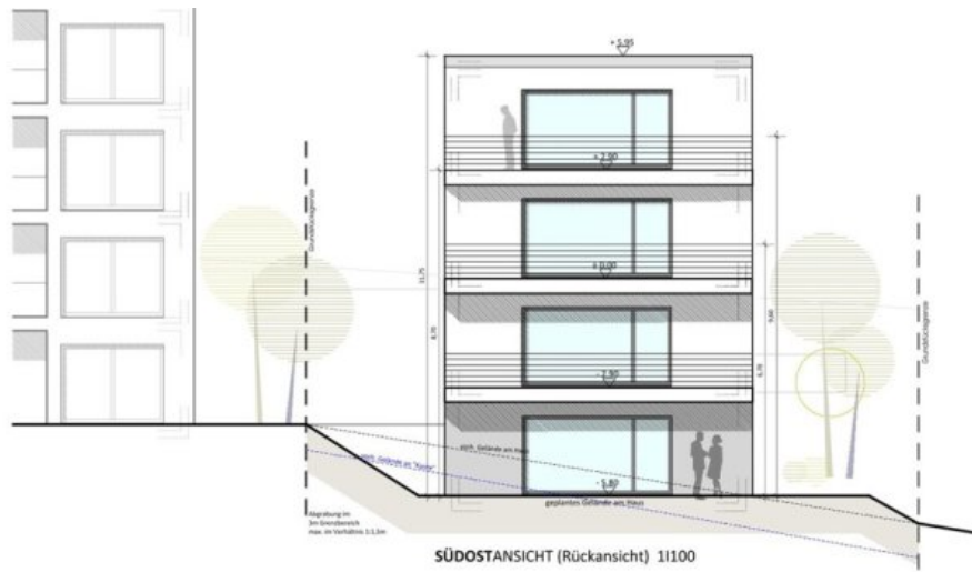
Rückansicht
