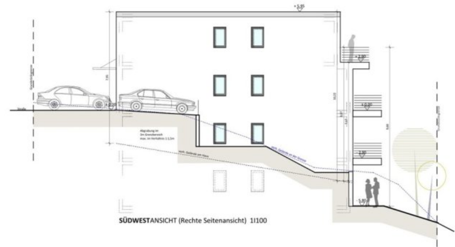
Südwestansicht
